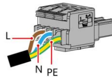
Klemme auf Wechselrichterseite (einphasig)
