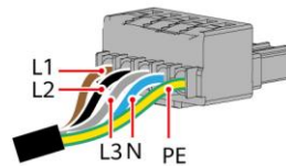
Klemme auf Wechselrichterseite (dreiphasig)
