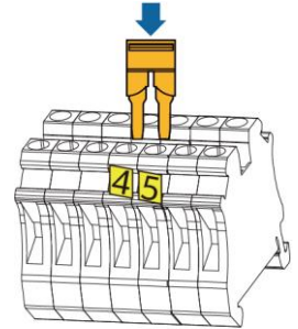
Netz-AC-Klemme X2 (einphasig/dreiphasig)
