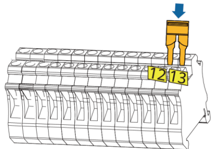
Wechselrichter-AC-Klemme X3 (dreiphasig)
